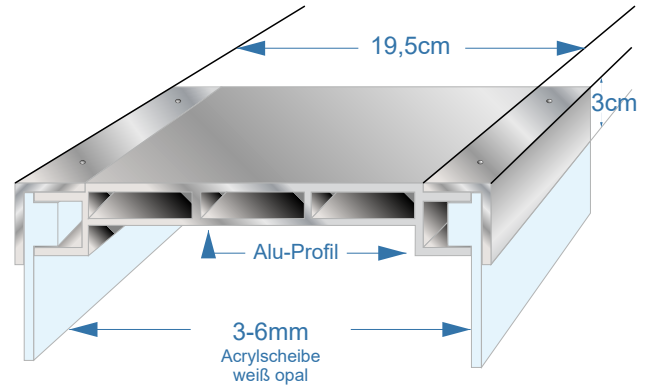
Profil Skizze Ausleger Scheibe
